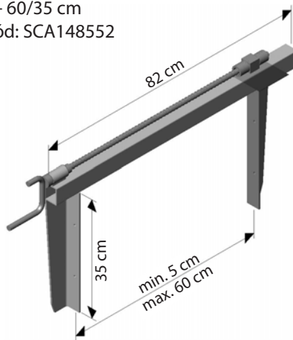
Bednicí svěrka
