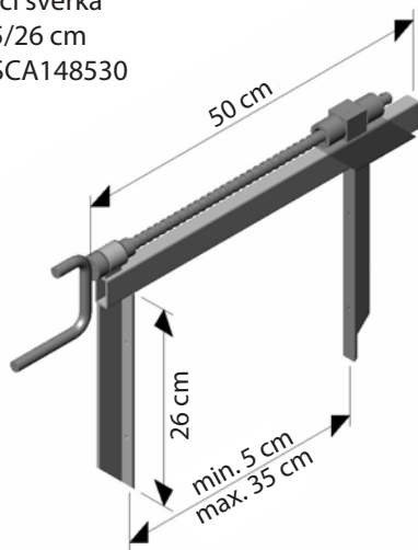
Bednicí svěrka
